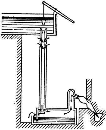
FIG. 108.—The trompe.
